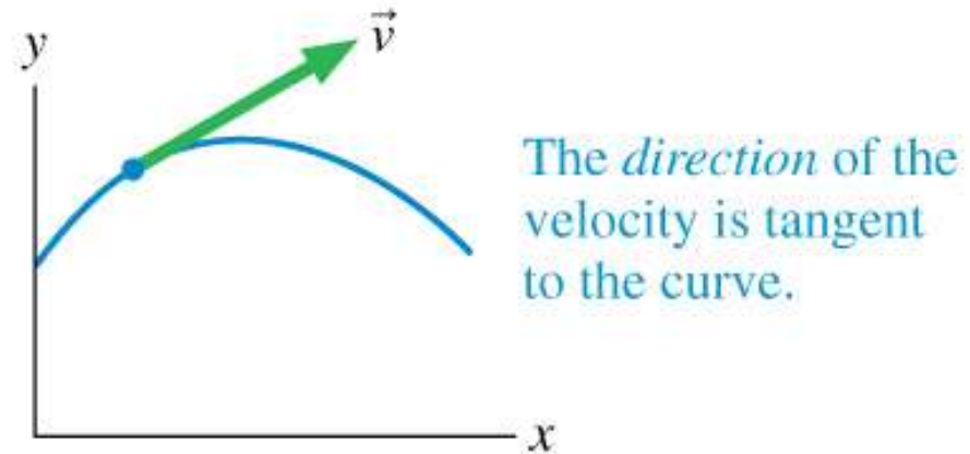
Trajectory
